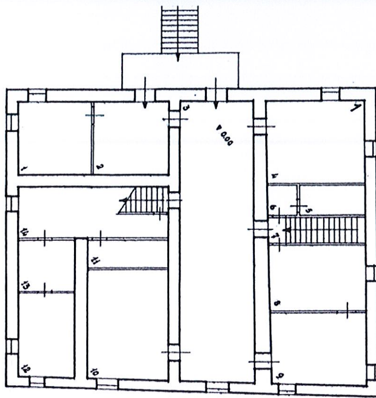
Piano Terra _ scala 1:200
